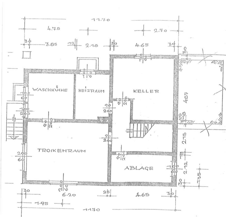
KELLERGESCHOSS, 1:100.
