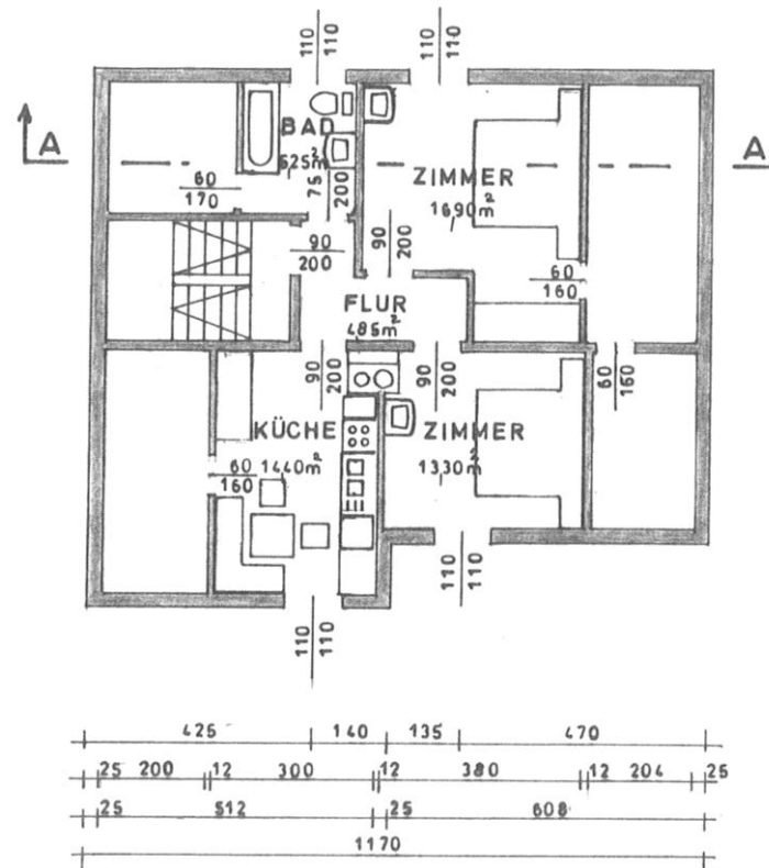
DACHGESCHOSS M 1-100
